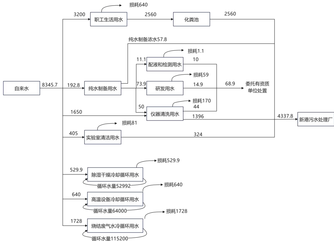
图2-1 水平衡图
