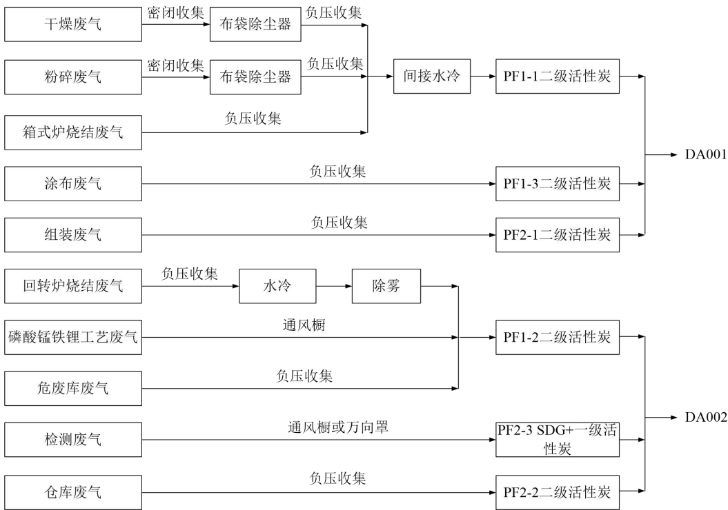
图6.1-1 废气收集路线图
