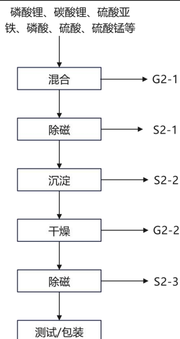
图 2-3 磷酸锰铁锂材料研发工艺流程及产污环节图（G 废气、S 固废、W 废水）
