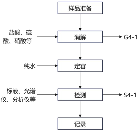
图 3.2-4 材料分析检测工艺流程及产污环节图（G 废气、S 固废、W 废水）
