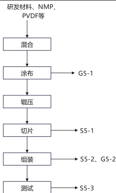
图 2-6 扣电/软包检测工艺流程及产污环节图（G 废气、S 固废、W 废水）
