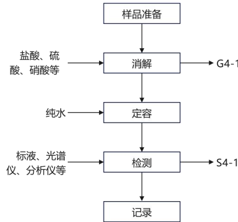
图 2-5 材料分析检测工艺流程及产污环节图（G 废气、S 固废、W 废水）
