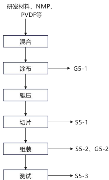
图 3.2-5 扣电/软包检测工艺流程及产污环节图（G 废气、S 固废、W 废水）
