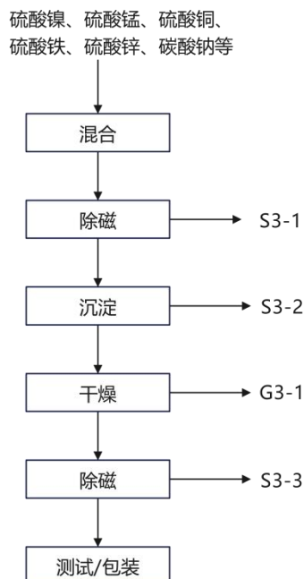
图 2-4 层状氧化物材料研发工艺流程及产污环节图 (G 废气、S 固废、W 废水)
