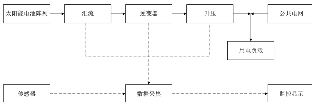
图 4-1 光伏发电工艺流程图
