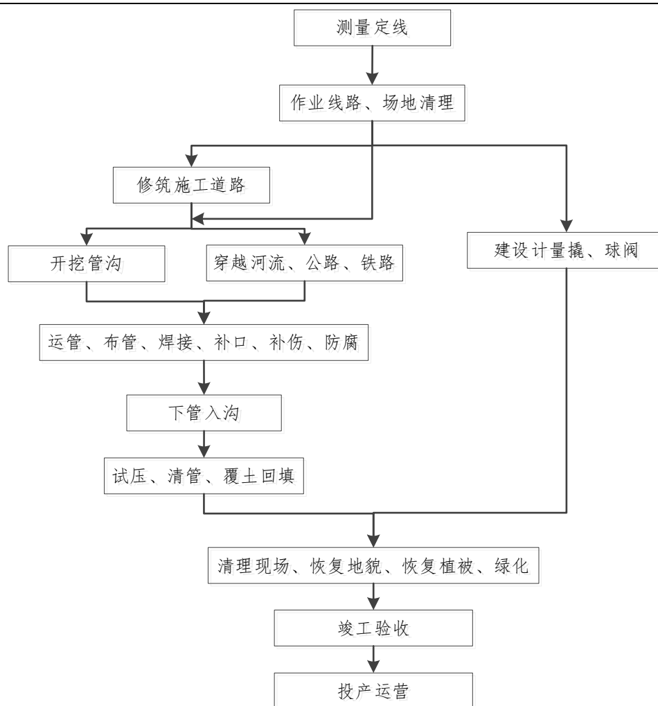
图 2-1 管道工程施工流程图
