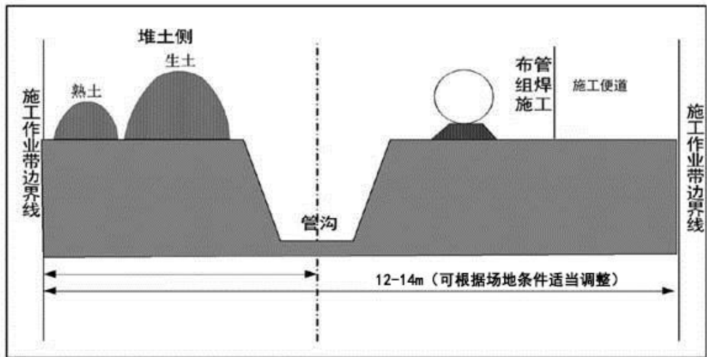
图 2-2 管沟作业带横断面布置示意图
