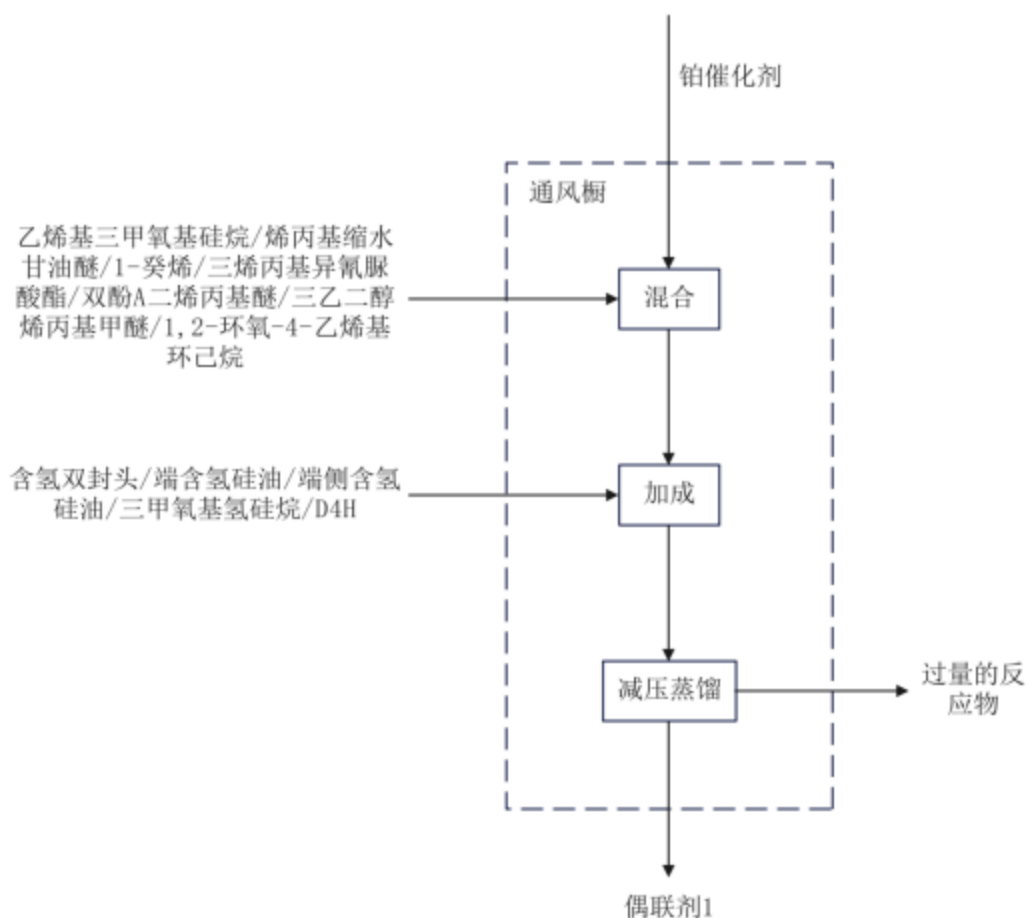
图 2-3 偶联剂 1 研发流程及产污环节
