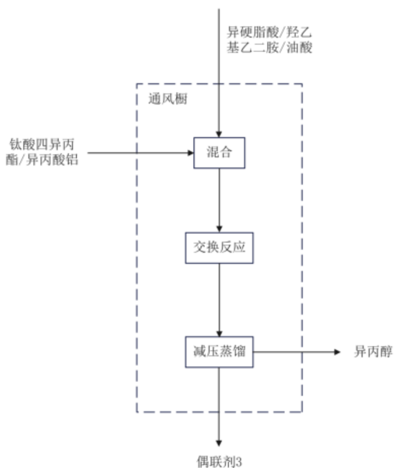
图 2-5 偶联剂 3 研发流程及产污环节
