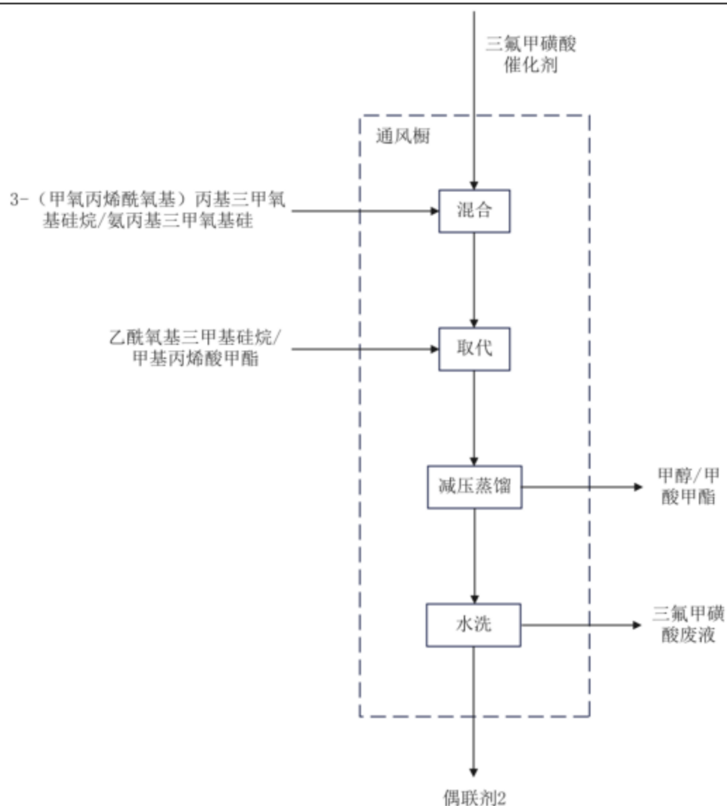
图 2-4 偶联剂 2 研发流程及产污环节
