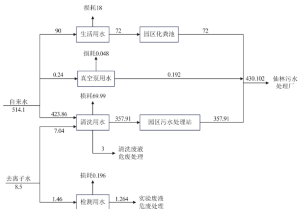
图 2-2 改建后企业水平衡图 单位: t/a
