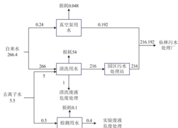
图 2-1 水平衡图 单位: t/a
