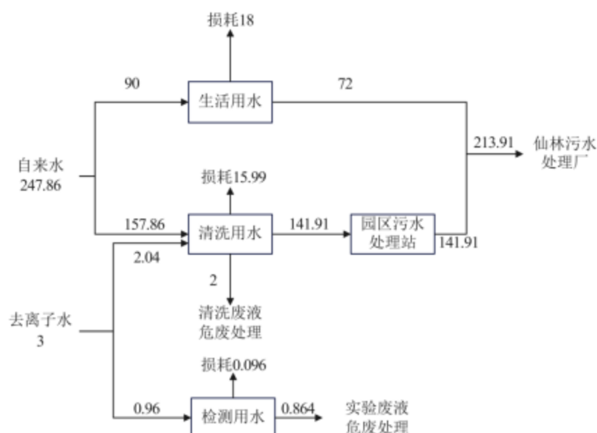
图 2-6 现有项目改建后水平衡图 单位：t/a
