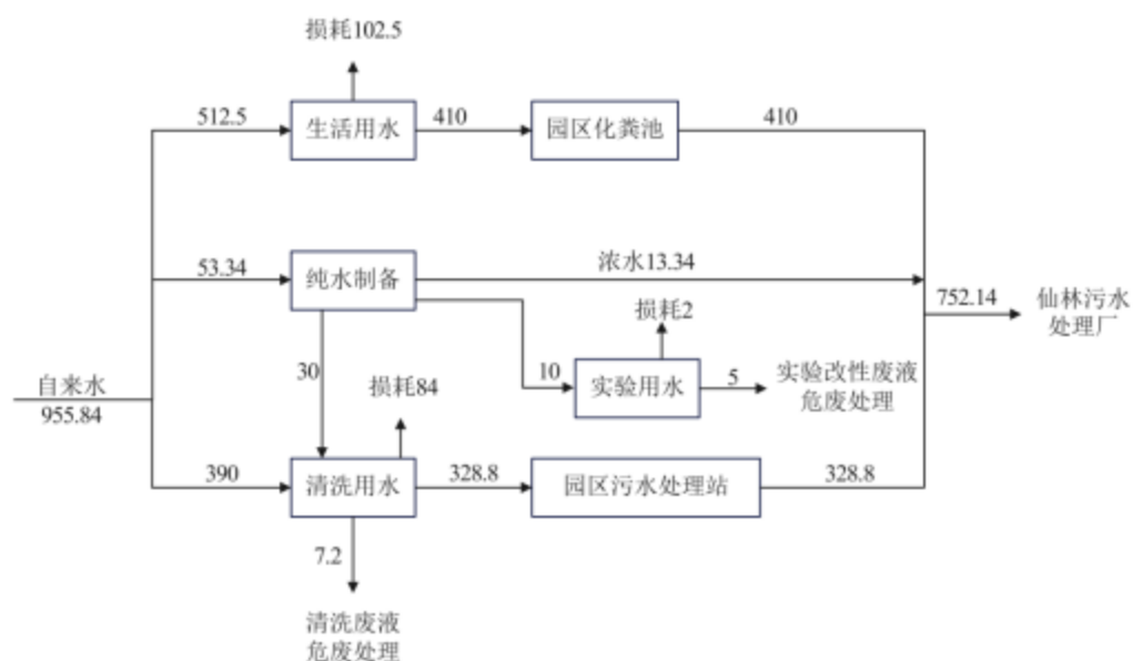
图 2-2 扩建后水平衡图 单位: t/a
