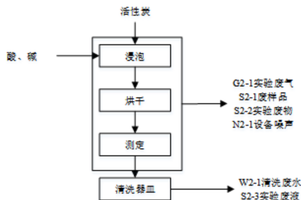
图 2-3 研发流程及产污环节
