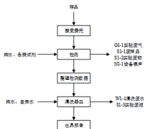
图 2-2 检测流程及产污环节
