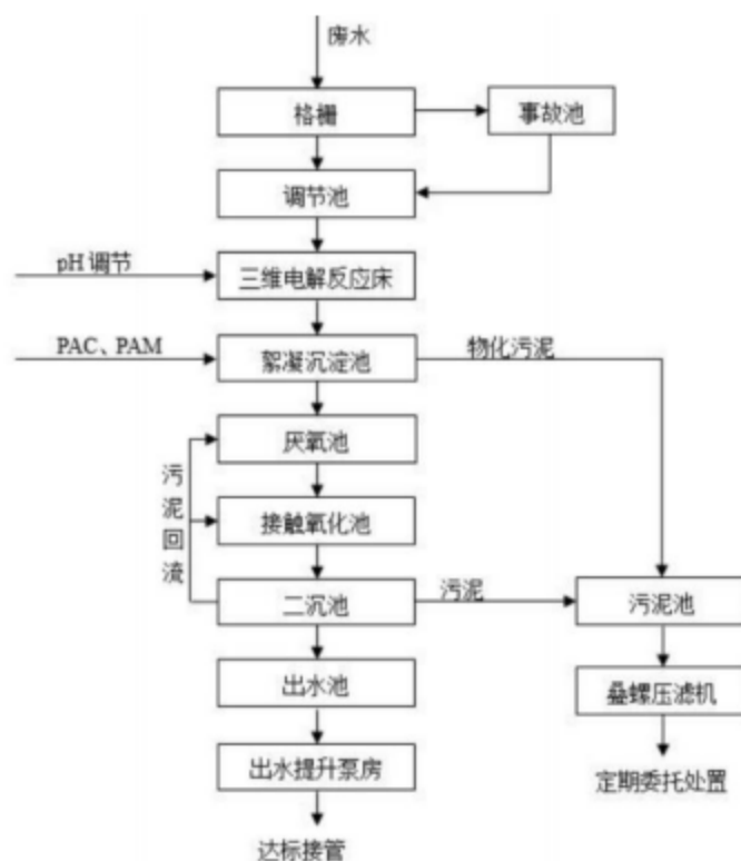
图 4-3 园区污水处理站工艺流程
