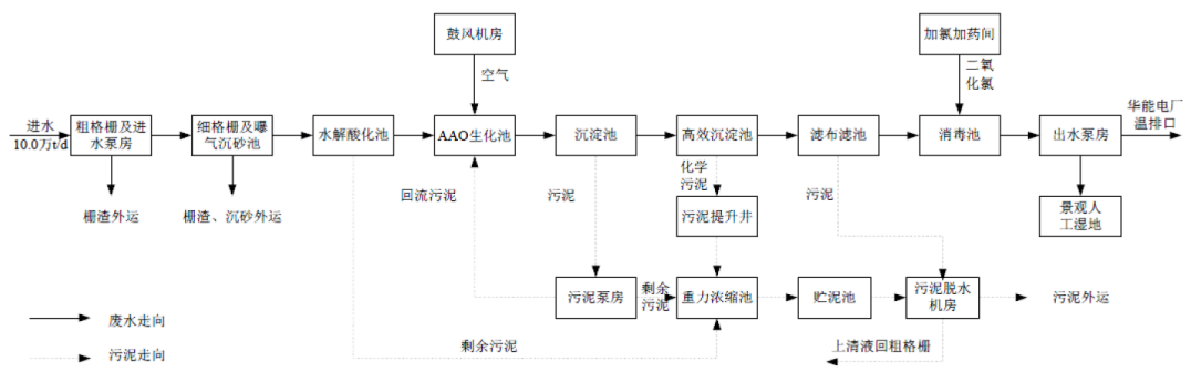
图4-2 南通市东港排水有限公司三期工艺流程图
